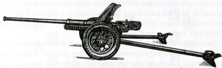
2 – 45-мм противотанковая пушка, образца 1937 г.
